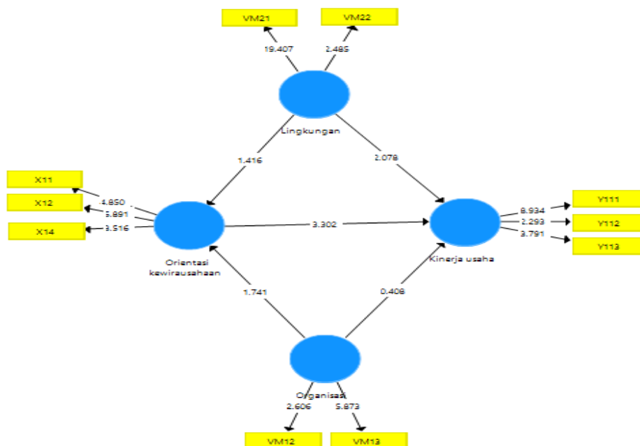
Gambar 2 model dengan nilai uji-t
